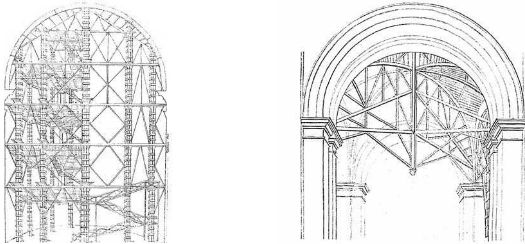
Fig.68-69 Basilica di Santa Maria degli Angeli: ponteggi per la ricostruzione del coro e della navata sinistra della basilica crollata per il terremoto del 1832. Progetto di Luigi Poletti, disegni di D.Bartoccini (Archivio della Porziuncola, 1832-35).
