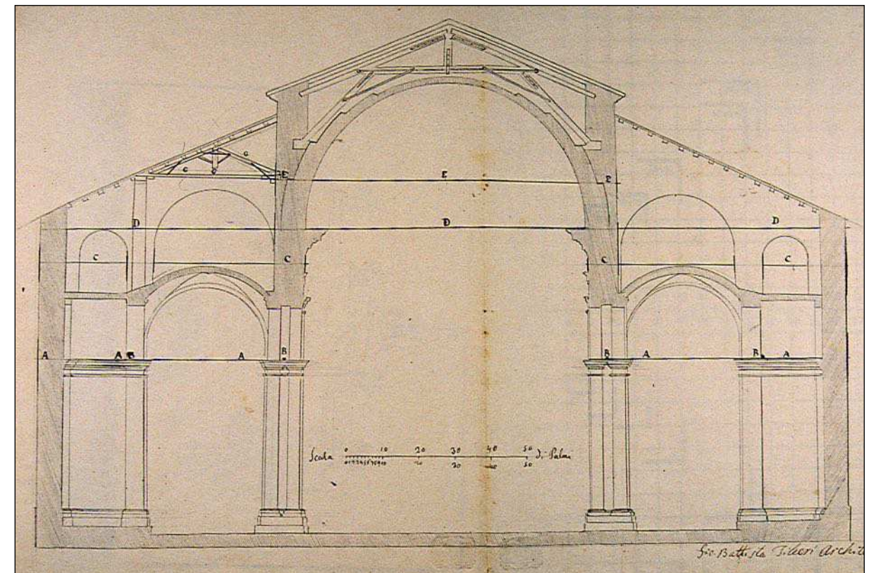
Fig.75-76 Basilica di Santa Maria degli Angeli: sezione trasversale e pianta disegnate da Giovanni Battista Tiberi, dopo il terremoto del 1854, con le indicazioni dei tiranti di rinforzo da collocare nell'edificio (Archivio della Porziuncola di Santa Maria degli Angeli, Carte sciolte , 20 ottobre 1855).
