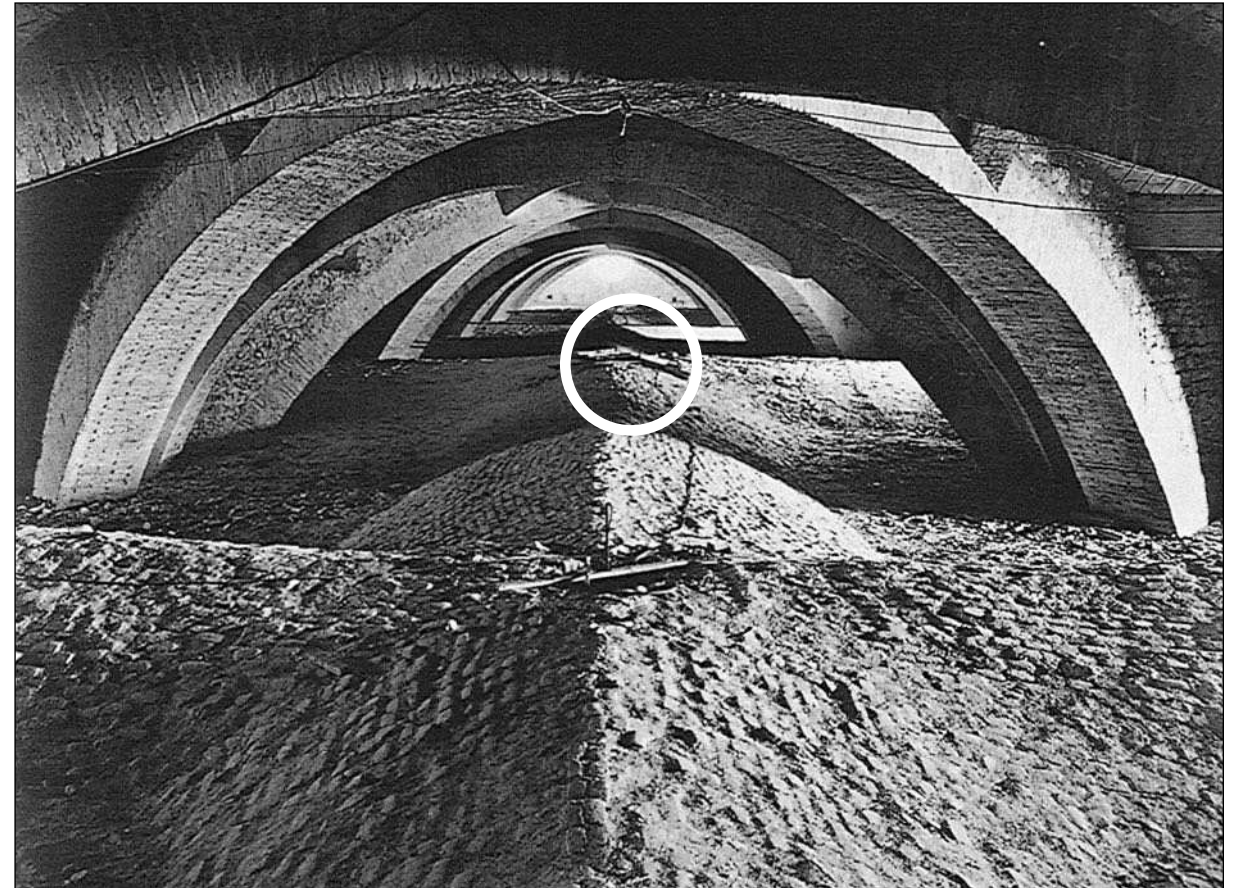
Fig.59 Assisi, basilica superiore di San Francesco, sottotetto della navata centrale (da Rocchi 1982): in primo piano, evidenziato con il cerchio bianco, è visibile un intervento di "cucitura" dell'arco dell'ultima volta della navata centrale, probabilmente fatto dopo il terremoto del 1832.
