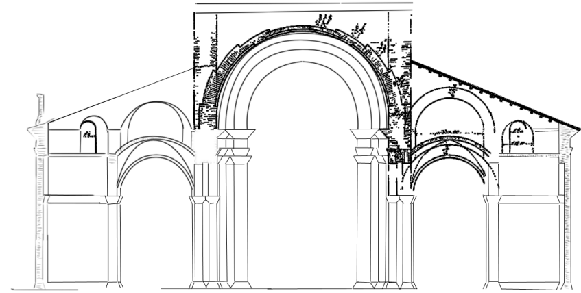
Fig.70 Basilica di Santa Maria degli Angeli: sezione trasversale disegnata da Luigi Poletti, dopo il terremoto del 1832, con le indicazioni per la rimodellazione degli archi (Biblioteca Civica di Stori dell'arte "Luigi Poletti" di Modena, Fondo Poletti).
