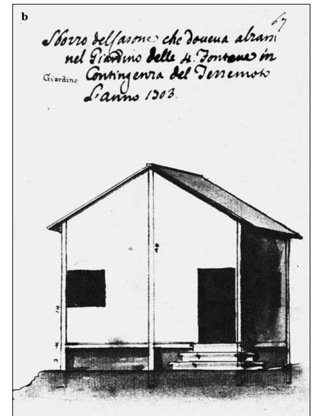
Fig.27 a e b Pianta e alzato di una casetta per ripararsi dal terremoto progettata a Roma in seguito alle numerose scosse avvenute nei primi mesi del 1703 (Biblioteca Apostolica Vaticana, cod. Barberini Latini, 4336).
