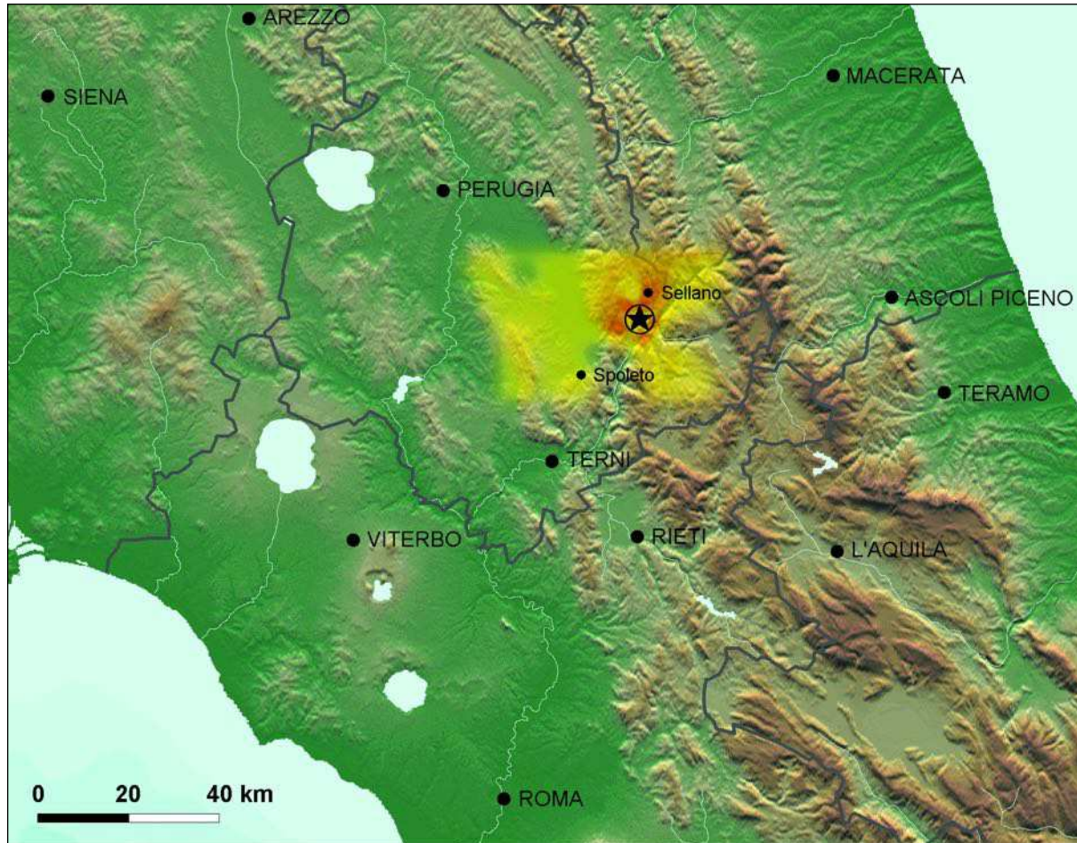
Fig.72 14 febbraio 1838: localizzazione dell'epicentro e degli effetti più gravi.
