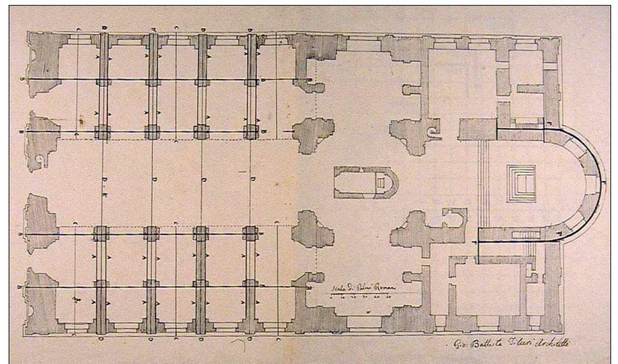
Fig.75-76 Basilica di Santa Maria degli Angeli: sezione trasversale e pianta disegnate da Giovanni Battista Tiberi, dopo il terremoto del 1854, con le indicazioni dei tiranti di rinforzo da collocare nell'edificio (Archivio della Porziuncola di Santa Maria degli Angeli, Carte sciolte , 20 ottobre 1855).
