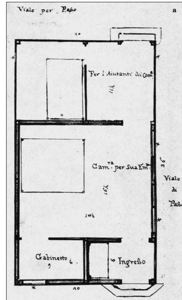
Fig.27 a e b Pianta e alzato di una casetta per ripararsi dal terremoto progettata a Roma in seguito alle numerose scosse avvenute nei primi mesi del 1703 (Biblioteca Apostolica Vaticana, cod. Barberini Latini, 4336).
