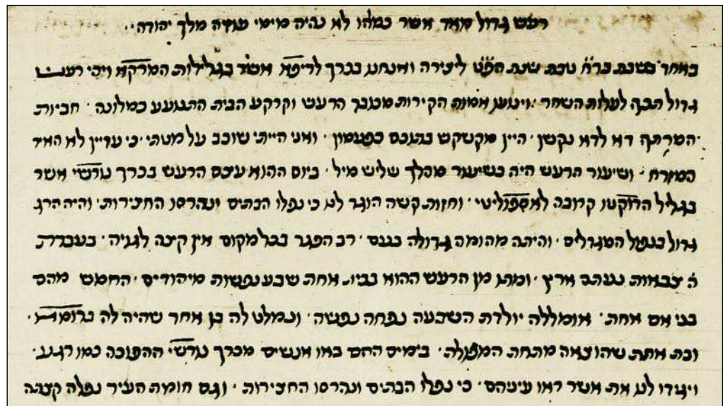
Fig.17 Particolare del "Libro di preghiere" di Moisé Ben Daniel (secolo XIV), in cui sono ricordati gli effetti del terremoto del 1328 a Norcia e a Ripatransone (Jewish National and University Library of Jerusalem, Heb. 8.o 4281).
