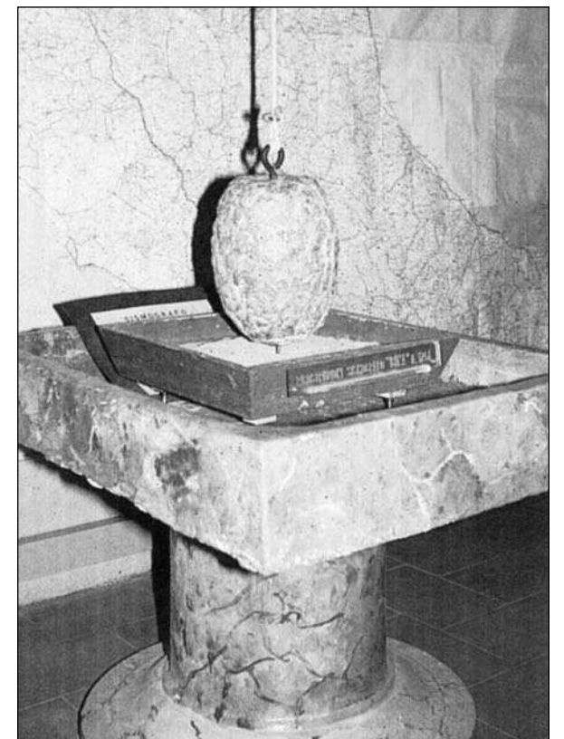
Fig.38 Osservatorio Sismologico di Perugia, presso l'Abbazia di San Pietro: ricostruzione del sismoscopio a pendolo di Andrea Bina.
