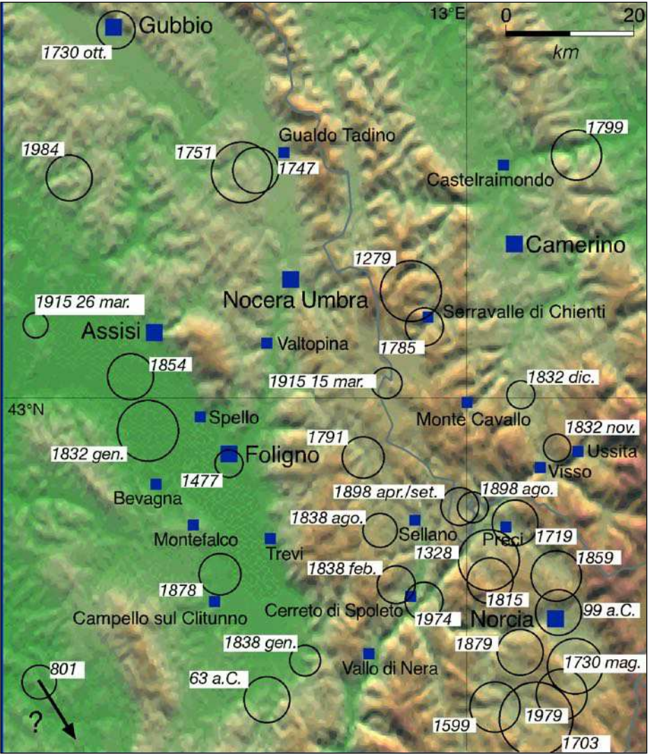
Fig.7 Terremoti dell'Appennino umbro-marchigiano analizzati in questo libro. Ogni terremoto è rappresentato mediante un simbolo circolare proporzionale alla magnitudo valutata a partire dai dati d'intensità (si veda il catalogo alla pagina seguente).
