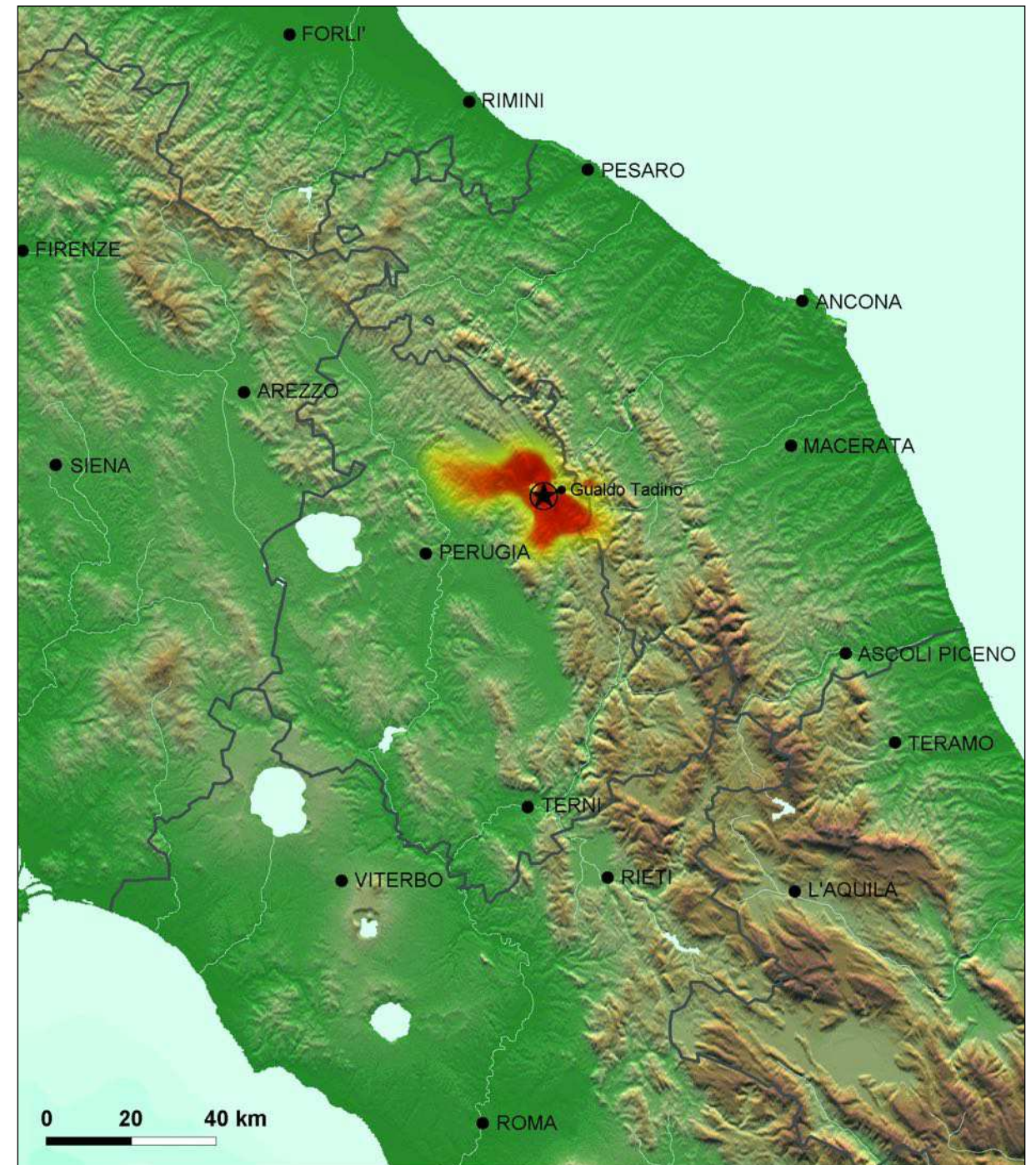
Fig.35 27 luglio 1751: localizzazione dell'epicentro e degli effetti più gravi.
